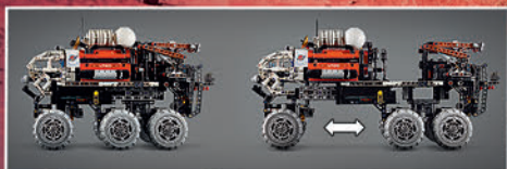
42180 Verkenningrover op Mars Vanaf 11 jaar
